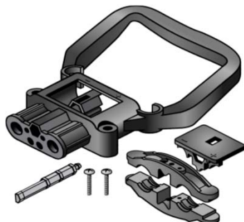
Lehrgehäuse Dose m. ang. HG, inkl. Zugentlasung und Verschlussstück
